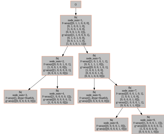
(d) Visualization of 6-D in FK-A
